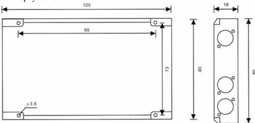
Тип корпуса: "O"
