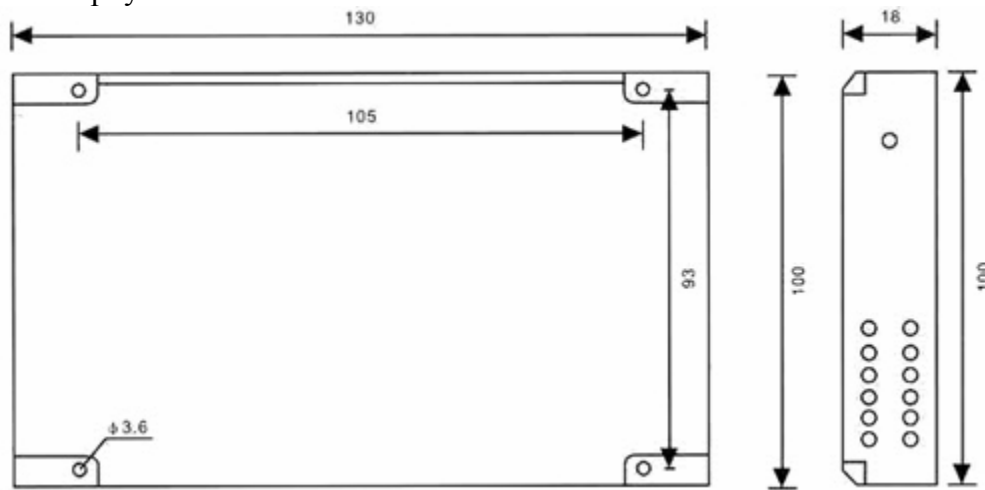
Тип корпуса: "L"
